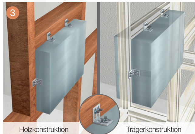
Auf der Rückseite mit den integrierten Edelstahl-Bolzen, die Box mittels Montagewinkeln an der Konstruktion befestigen.
